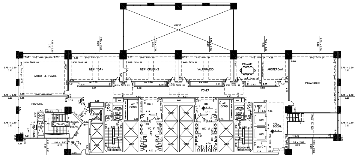
PLANTA DO PAVIMENTO C1 Esc. 1:100
